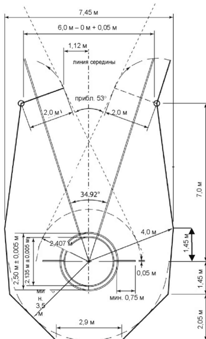
Рисунок (а) ТПЗ7 - заградительный сектор для метания молота и диска с концентрическими кругами (расположение для метания молота для праворукого метателя с указанием размеров заградительного сектора до сетки)
