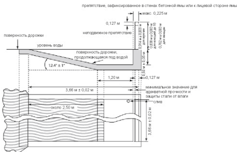
Рисунок (б) ТП23 - Яма с водой
