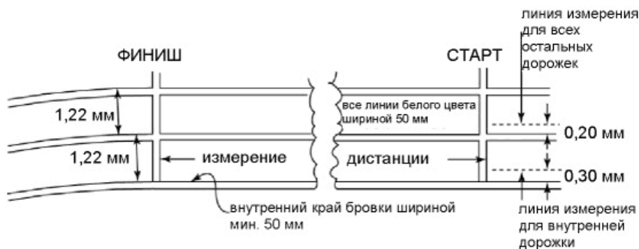
Рисунок ТП14 - Измерения дорожки (вид со стороны первой дорожки)
