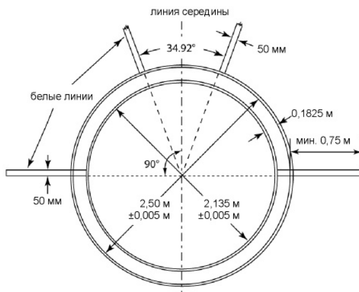
Рисунок (д) ТП32 - схема концентрических кругов для метания диска и молота
