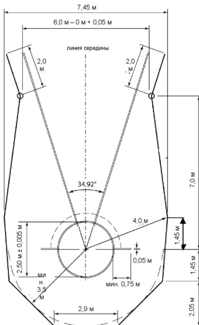
Рисунок (б) ТПЗ7 - заградительный сектор для метания молота и диска с концентрическими кругами (конфигурация для метания диска, с указанием размеров заградительного сектора до сетки)
