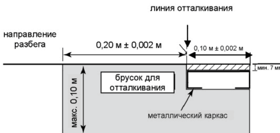
Рисунок (a1) ТП29 - брусок для отталкивания с заглушкой
