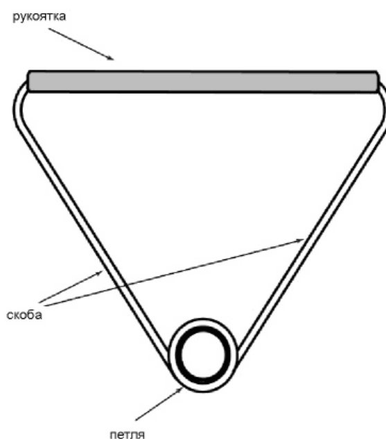
Рисунок (б) ТПЗ6 - универсальная рукоятка молота
