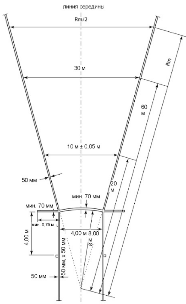
Рисунок (е) ТП32 - зона разбега и сектор для метания копья
