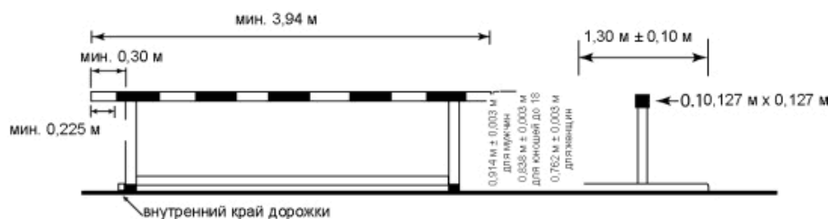
Рисунок (а) ТП23 - пример препятствия
